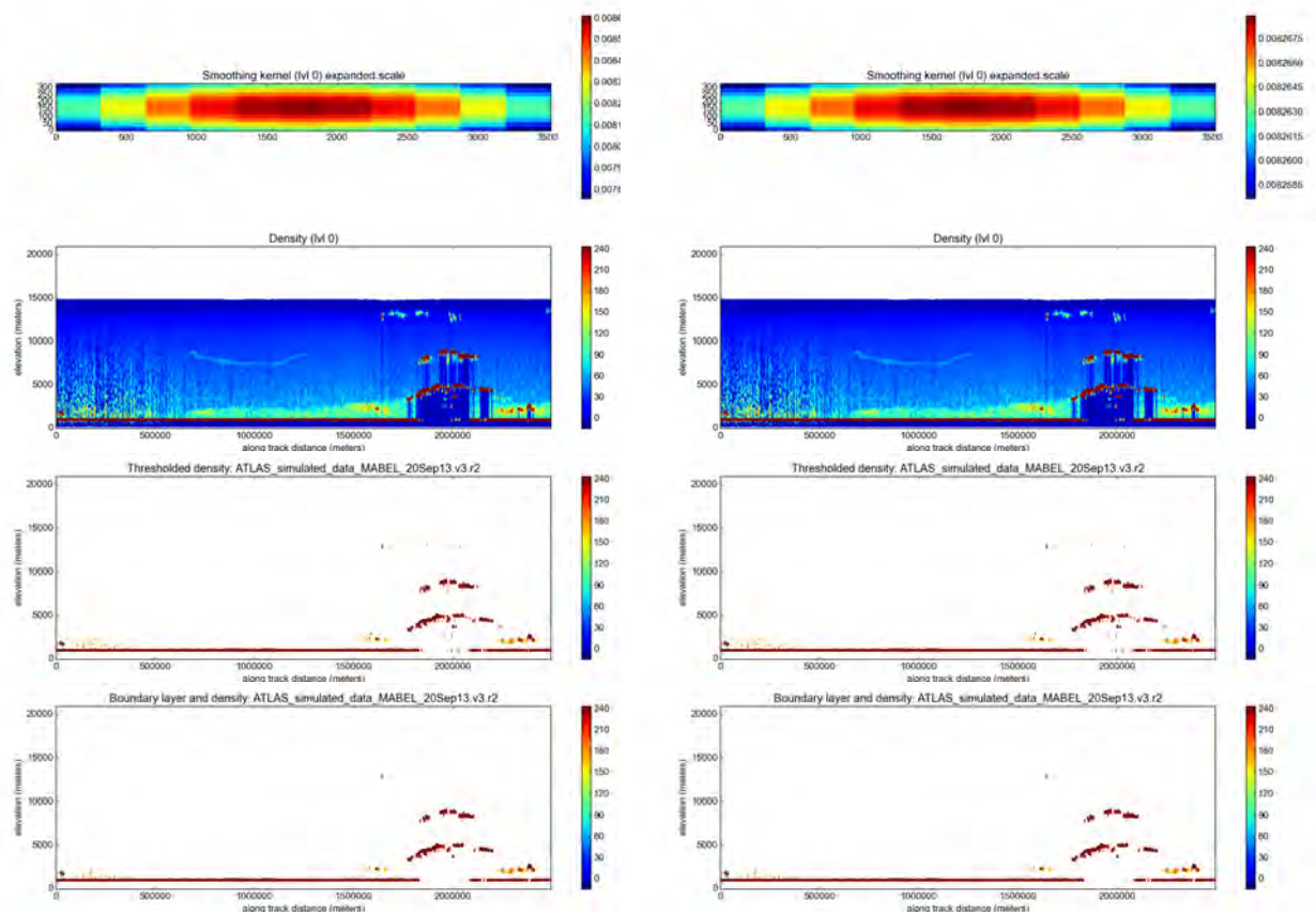
g) \sigma = 16
